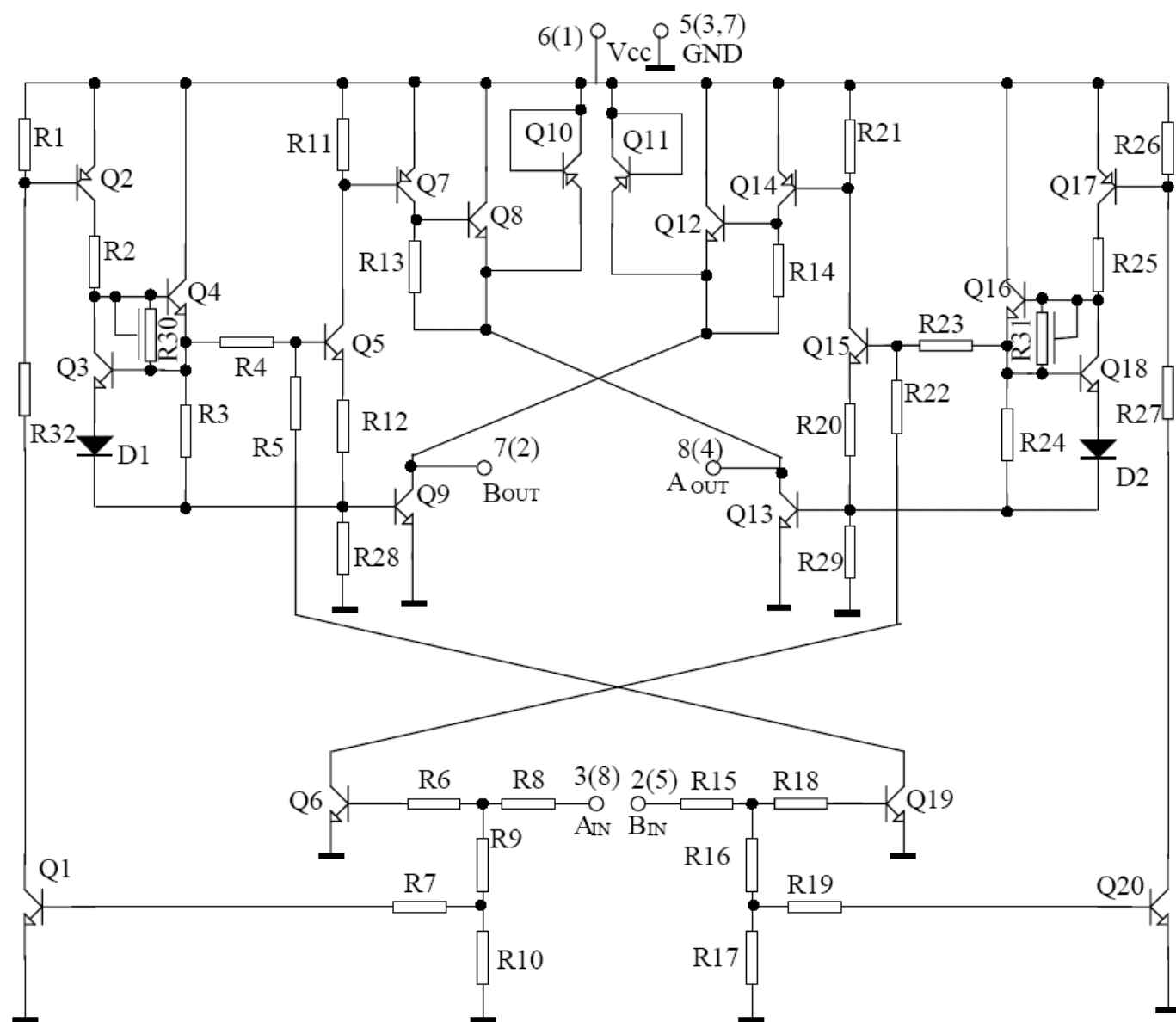
内部线路图
