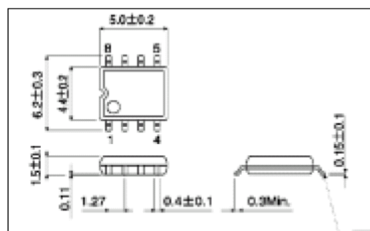
管脚排列图
