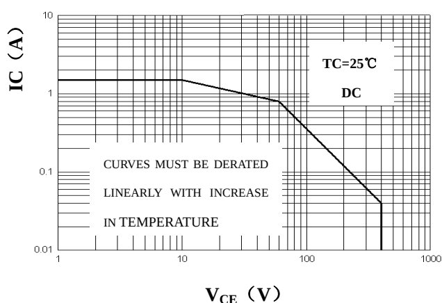
SOA
