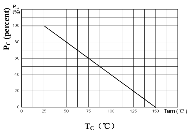
P_C - T_C
