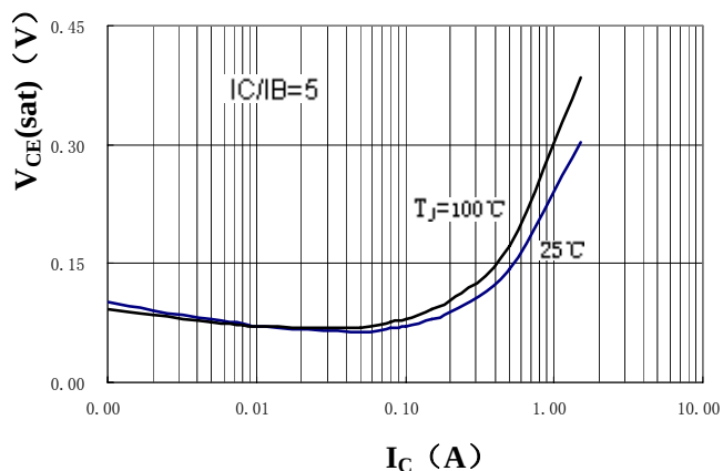
V_{CE(sat)} - I_C
